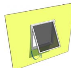
Figura 2.67. Ventana proyectante: 7.6 m^3/h m^2 Proyectante de doble contacto: 4.5 m^3/h m^2
