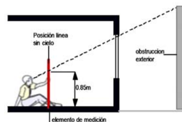
Figura 5.17. Medición línea sin cielo en un recinto.
