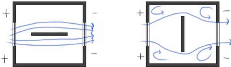
Figura 4.6. Ventilación afectada por muros interiores
