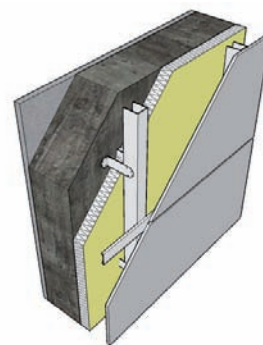
Figura 2.12. Solución Muro N° 3 Muro de hormigón armado de e : 200 mm. con estuco interior de e : 25 mm y sistema de fachada ventilada, con aislante térmico de lana de vidrio en rollo, en diferentes espesores, cámara de aire ventilada y revestimiento exterior en panel de fibrocemento.
