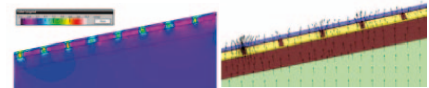
Figura 2.56. Detalle original complejo de techumbre. Flujo de calor y vectores. Escuela Monseñor Francisco Valdés Subercaseaux, Curarrehue. (Fuente: Informe técnico Thiele & Sommerhoff consultores)
