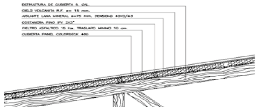
Figura 2.55. Detalle original complejo de techumbre. Escuel Escuela Monseñor Francisco Valdés Subercaseaux, Curarrehue. (Fuente: Informe técnico Thiele & Sommerhoff consultores)
