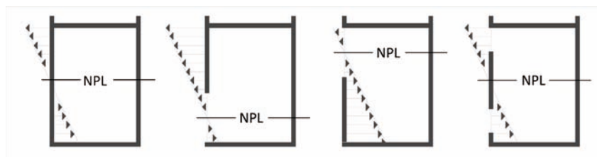
Figura 4.10. Diagramas en corte que ilustran los niveles de presión neutra (NPL) para distintas ubicaciones de vanos.
