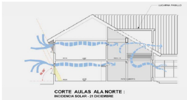
Figura 4.7. Estrategia de ventilación cruzada en la Escuela Teniente Merino de Cochrane (zona 8 SE), donde se puede observar que ventanas proyectantes entre las aulas y el pasillo facilitan el flujo de aire.
