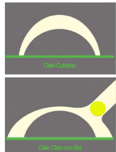
Figura 5.5. Esquema de distribución de luminancias cielo cubierto y cielo claro.
