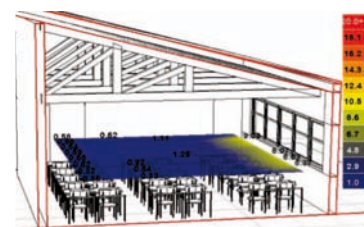
Figura 33. Simulación Lumínica sala de clases 7. Escuela Francisco Valdés Subercaseaux. Curarrehue, Región de la Araucanía.
