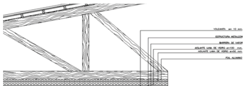
Figura 2.57. Detalle modificado complejo de techumbre. Escuela Monseñor Francisco Valdés Subercaseaux, Curarrehue. (Fuente: Informe técnico Thiele & Sommerhoff consultores)
