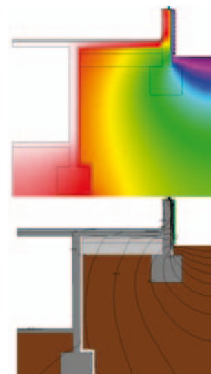
Figura 32. Simulación de puentes térmicos, detalle envoltente térmica fundación y muro perimetral piso 1 Edificio Policía de Investigaciones de Puerto Montt.
