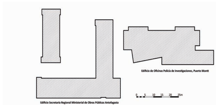
Figura 1.23. Sombra de planta Edificio Secretaría Regional Ministerial de Obras Públicas, Antofagasta, región de Antofagasta y Edificio de Oficinas Policía de Investigaciones, Puerto Montt Décima Región de los Lagos. Grafica cómo se buscó maximizar la superficie de envolvente al modificar la planta del edificio en Antofagasta y cómo el edificio en Puerto Montt busca una planta más compacta para disminuir su factor de forma.
