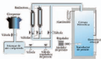
Figura 2.61. Esquema banco de ensayos de ventanas
