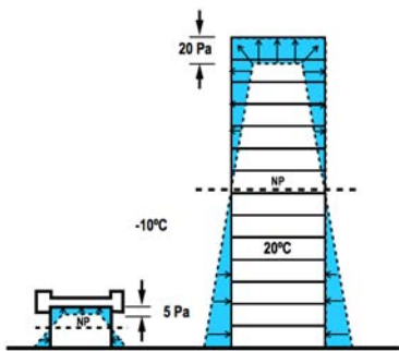
Figura 2.73. Figura 2. 3: Diferencias de presión producidas por diferencias de temperaturas.
