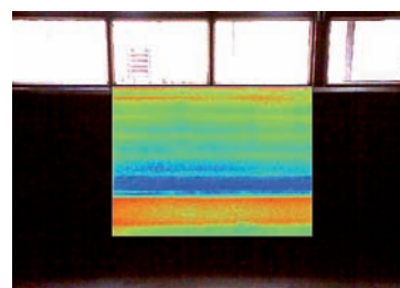
Figura 26. Imagen termográfica de envolvente. Escuela Rucamanke.
