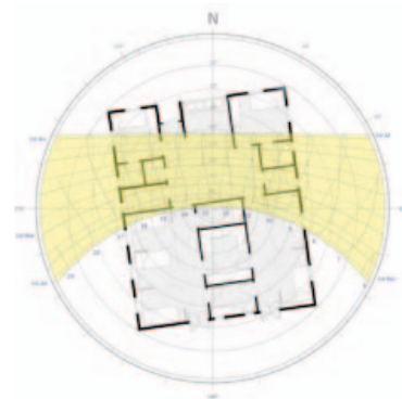
Figura 5.11. Diagrama Sun Path.
